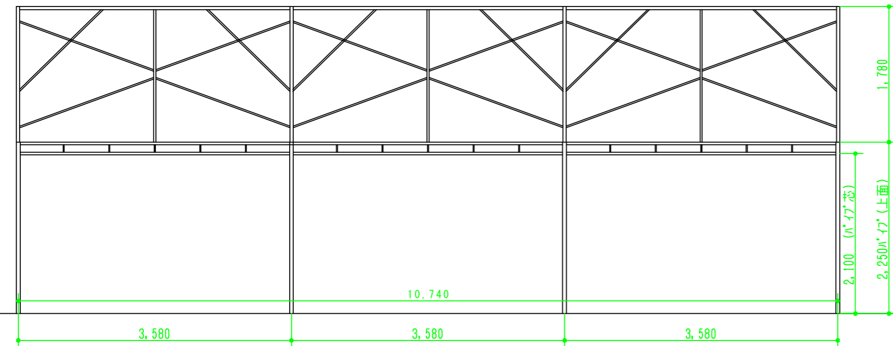
側面図
